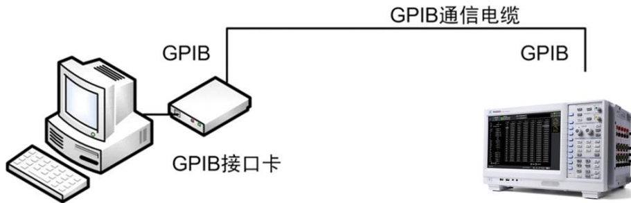
图 2.3 GPIB 硬件连接图
