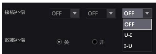
图 5.31 接线补偿方式的选择
