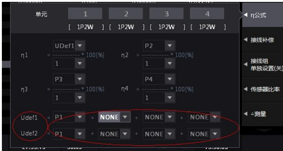
图 5.9 效率运算参数设定
