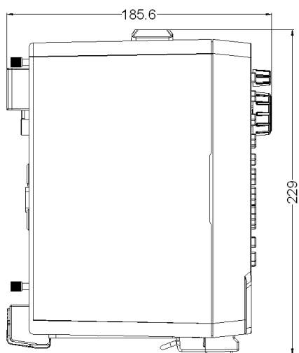
图 8.4 尺寸图 3
