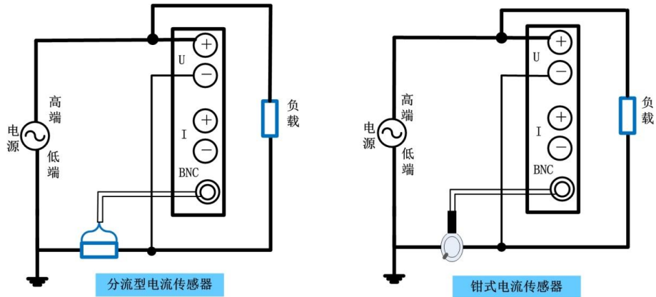
图 4.13 接线原理图
