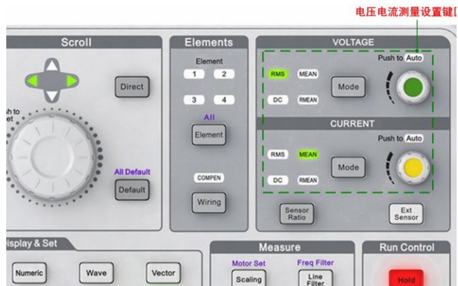
图 3.7 电压/电流测量设置键区
