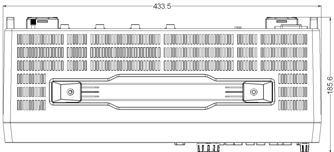
图 8.2 尺寸图 1
