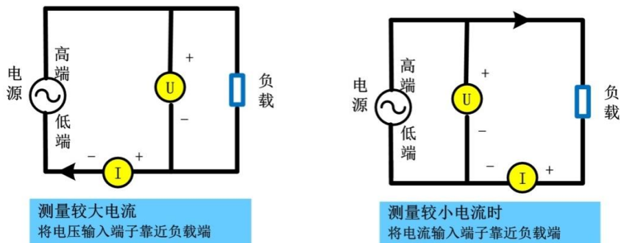
图 4.4 测量电压和电流的大小对测量的影响
