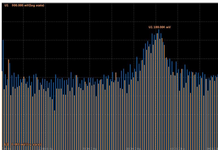
图 2.10 谐波/间谐波子组
