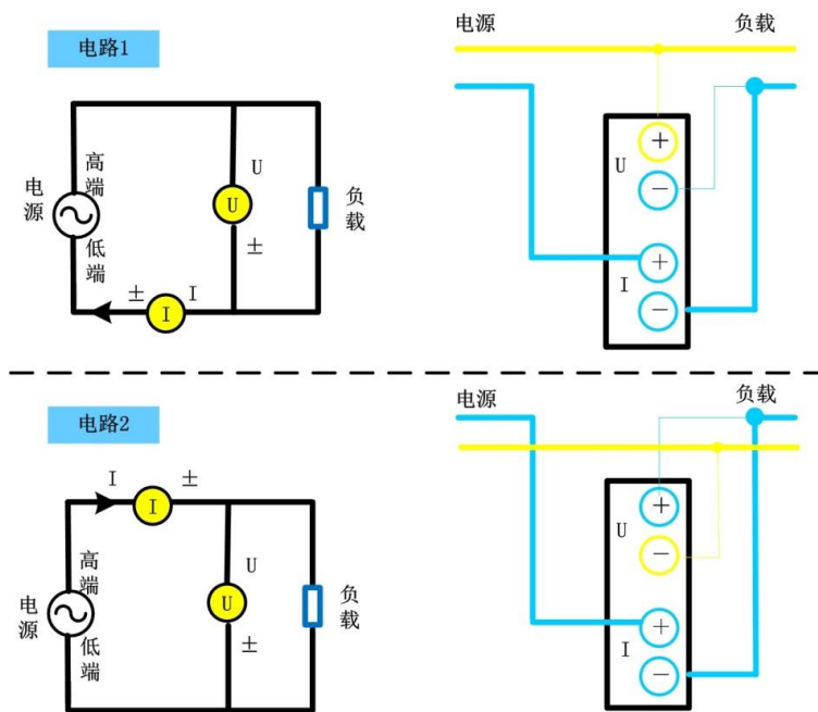
图 4.5 单相 2 线制(1P2W)，测量仪表的接线
