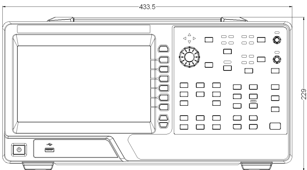
图 8.3 尺寸图 2
