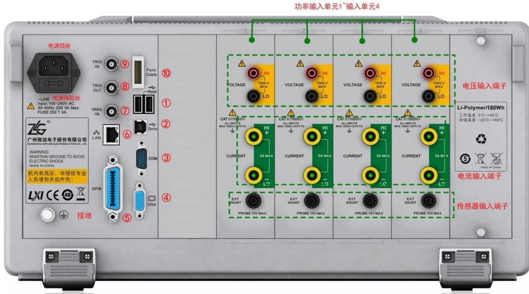
图 3.14 后面板说明
