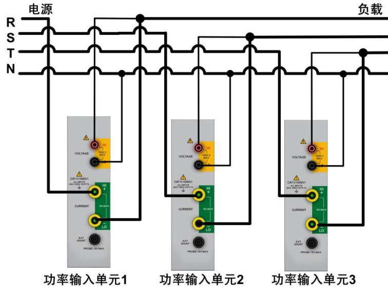
图 4.49 三相 4 线制接线实例
