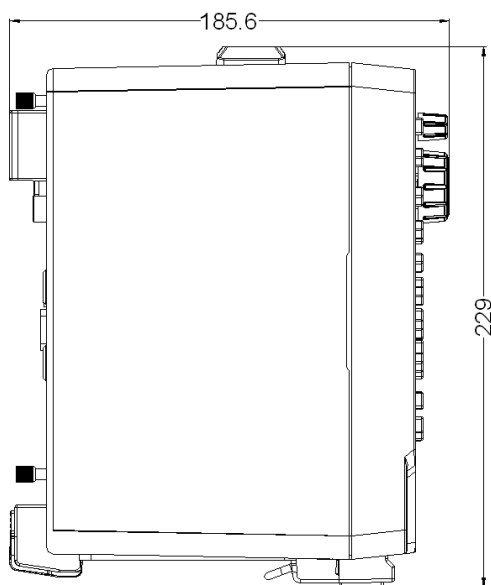
图 7.3 尺寸图 3
