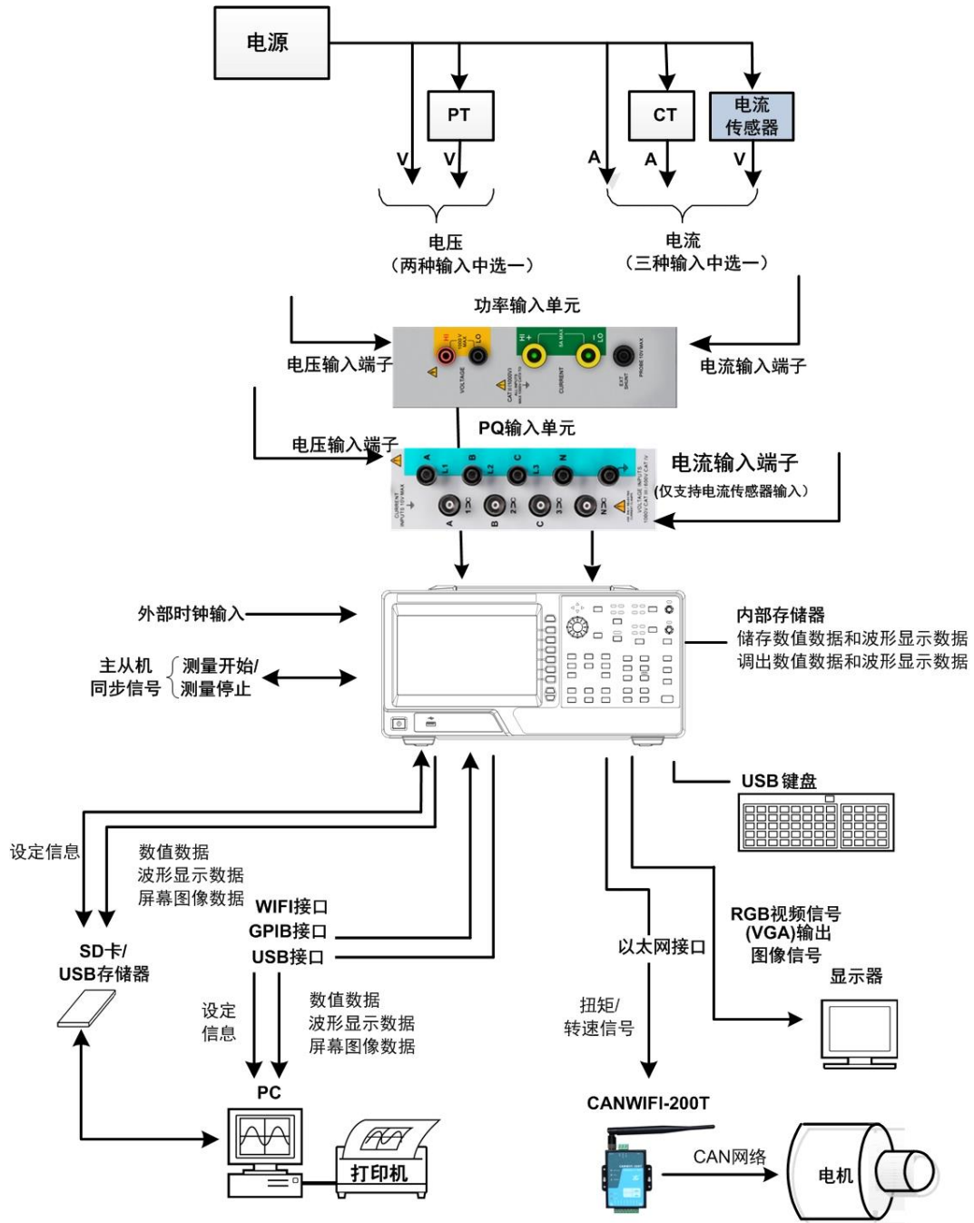
图 1.2 应用系统
