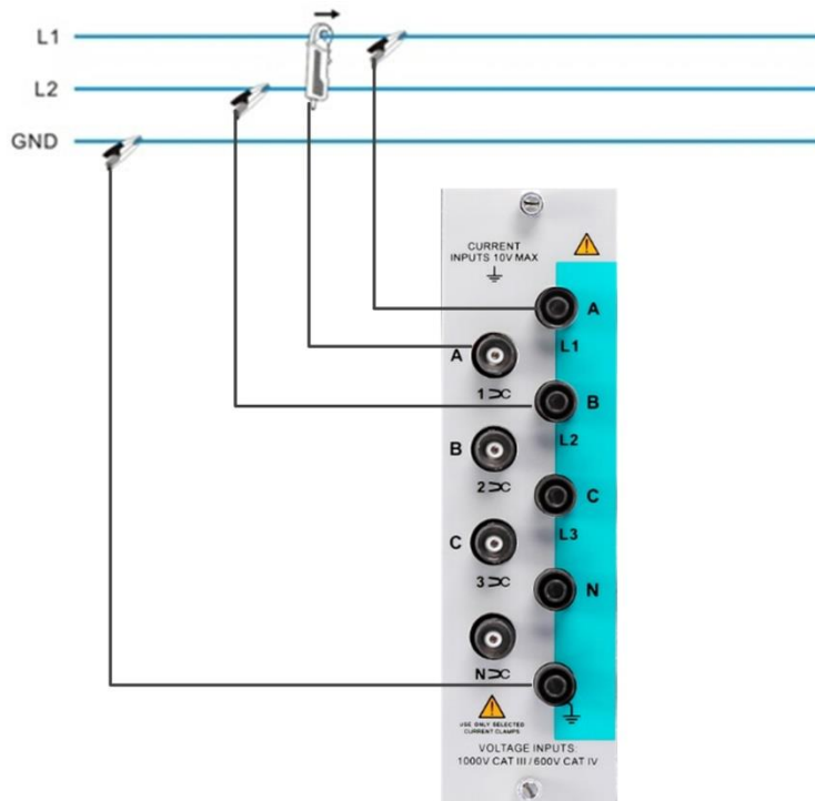
图 4.51 1P2W-No Neutral
