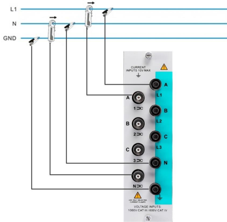
图 4.50 1P2W-Neutral
