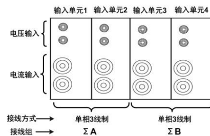
图 2.21 接线组
