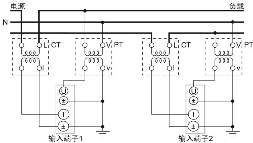
图 4.39 单相 3 线制(1P3W)、使用 PT/CT 时的接线举例
