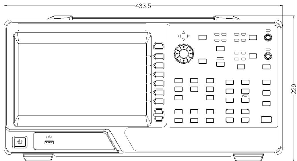
图 7.2 尺寸图 2
