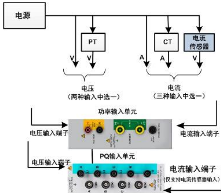
图 2.20 输入信号到输入单元
