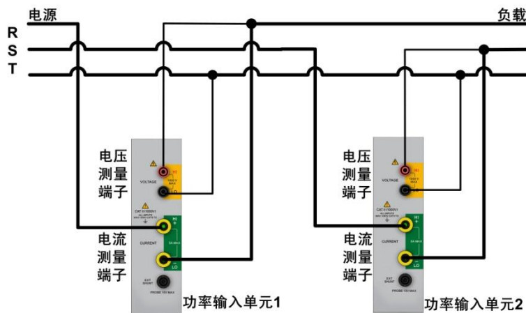
图 4.43 3P3W 下新能源汽车综合分析仪接线实例
