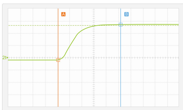
300V电压上升时间30.8us
