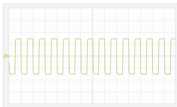
方波输出 (150V/2kHz)
