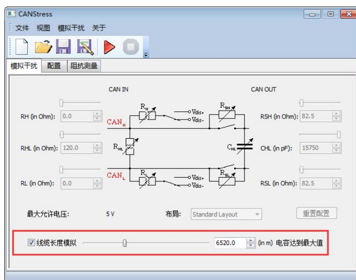
图 8.106 模拟导线长度
