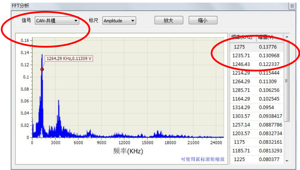
图 8.70 波形记录 FFT 分析
