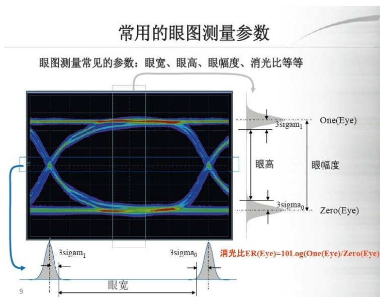
图 8.24 常用眼图测量参数
