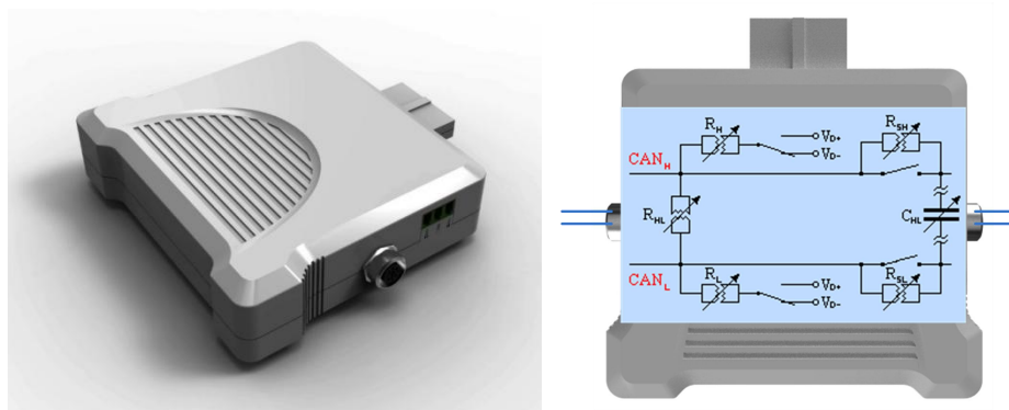
图 3.8 CANScope-StressZ 模拟测量与干扰扩展板（选配）
