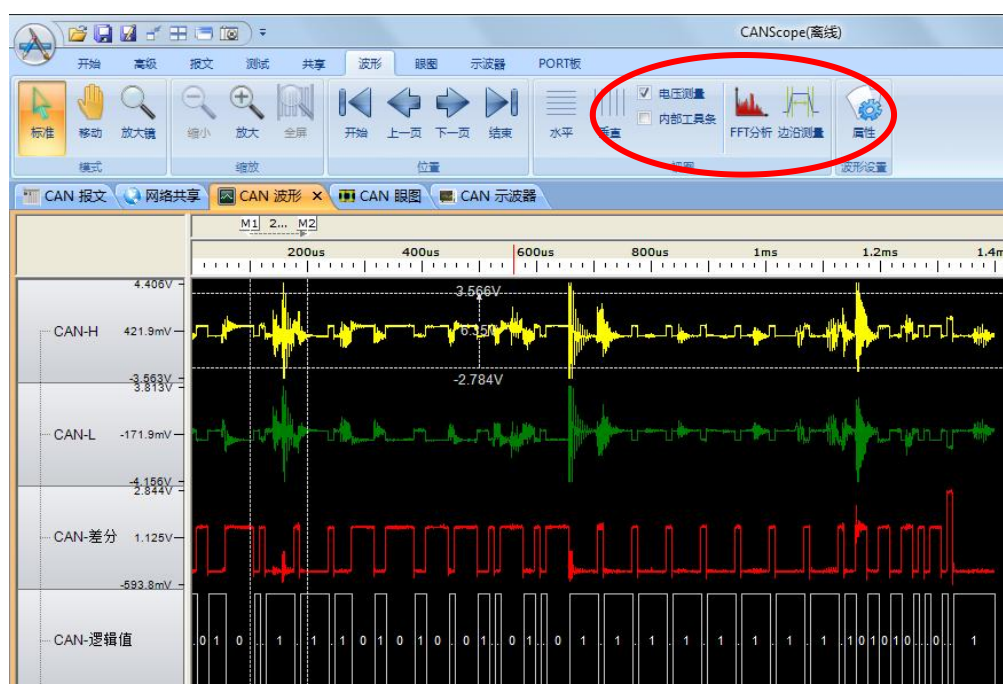
图 8.69 单帧 FFT 分析
