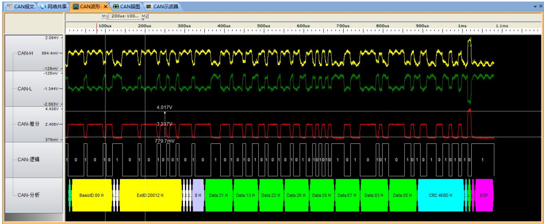
图 8.46 CAN 波形展示
