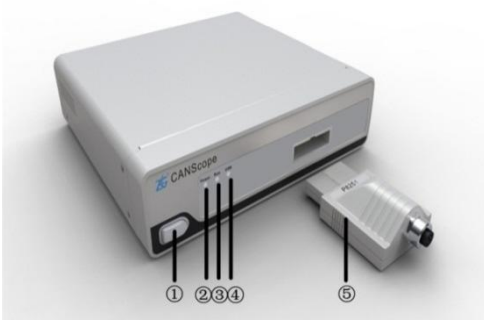
图 3.4CANScope 正面
