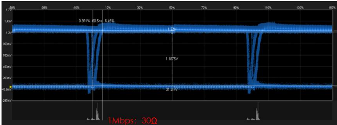
图 8.96 终端电阻过小
