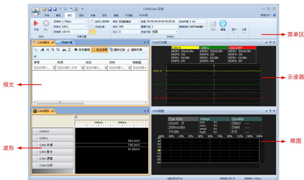
图 8.1 CANScope 主界面
