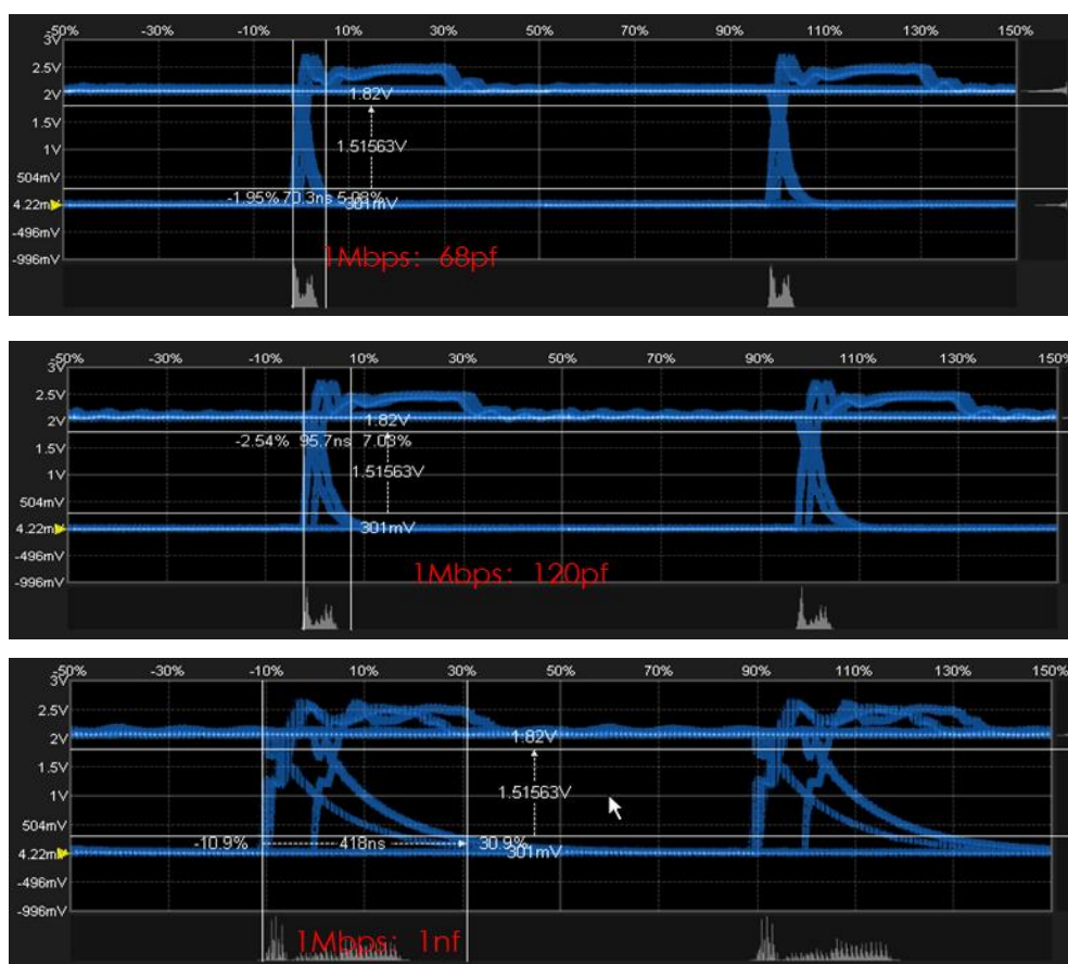
图 8.103 负载电容变化的眼图
