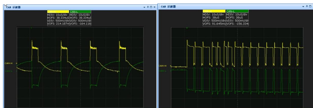
图 8.18 终端电阻不连接与连接的 CAN 总线波形对比
