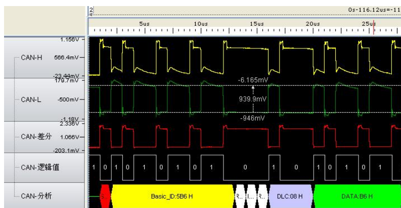
图 8.61CAN 波形_电压测量
