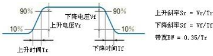
图 8.85 边沿区间
