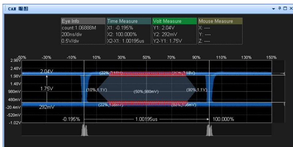
图 8.20 眼图分析
