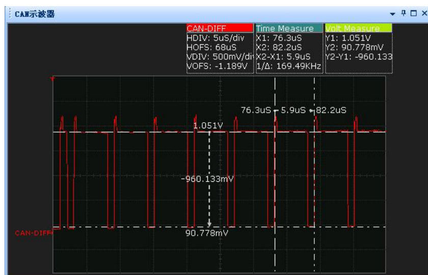
图 8.15CAN 示波器_时间测量和电压测量
