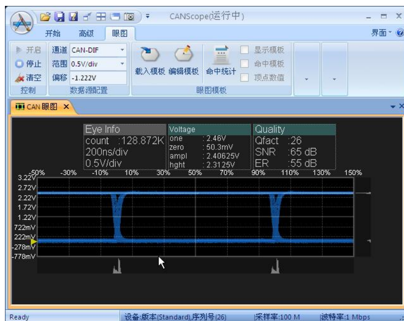
图 8.22CAN 眼图界面
