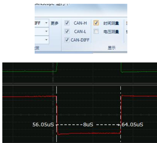
图 8.2 CAN 示波器上测量最小脉宽获得波特率
