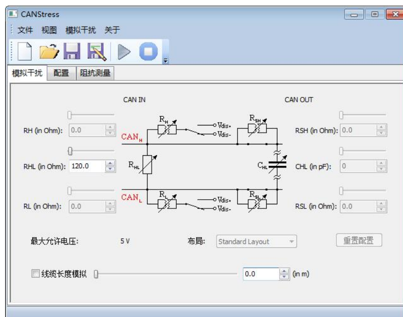
图 5.31 CANScope-StressZ 界面
