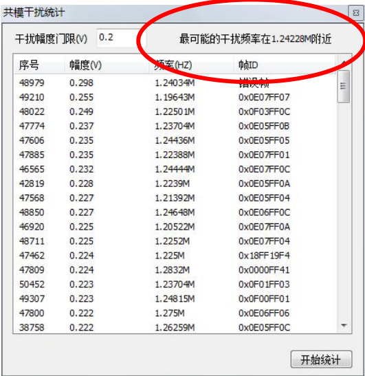
图 8.72 共模干扰统计结果
