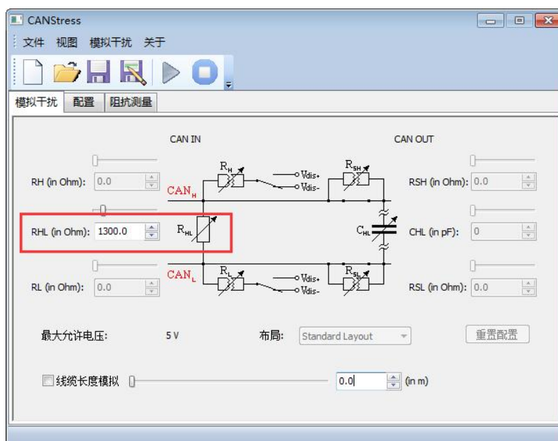
图 8.94“CANStress”窗口_配置 R HL 阻值为 1300 欧姆
