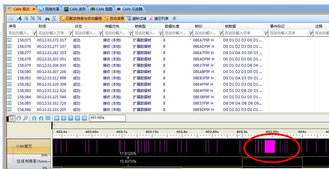
图 8.169 拥堵位置
