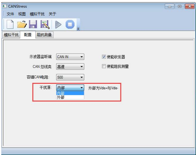
图 8.104 选择干扰源
