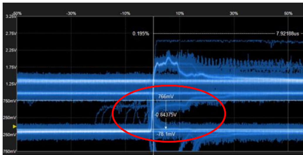
图 8.21 远距离传输的眼图
