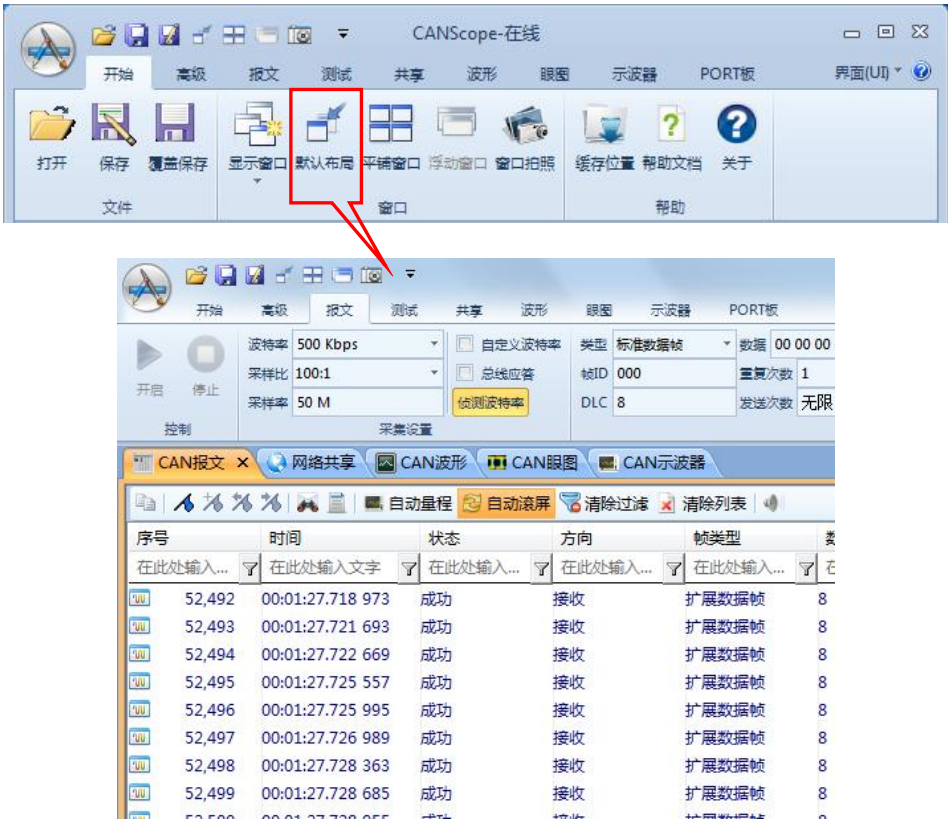
图 6.4 默认窗口
