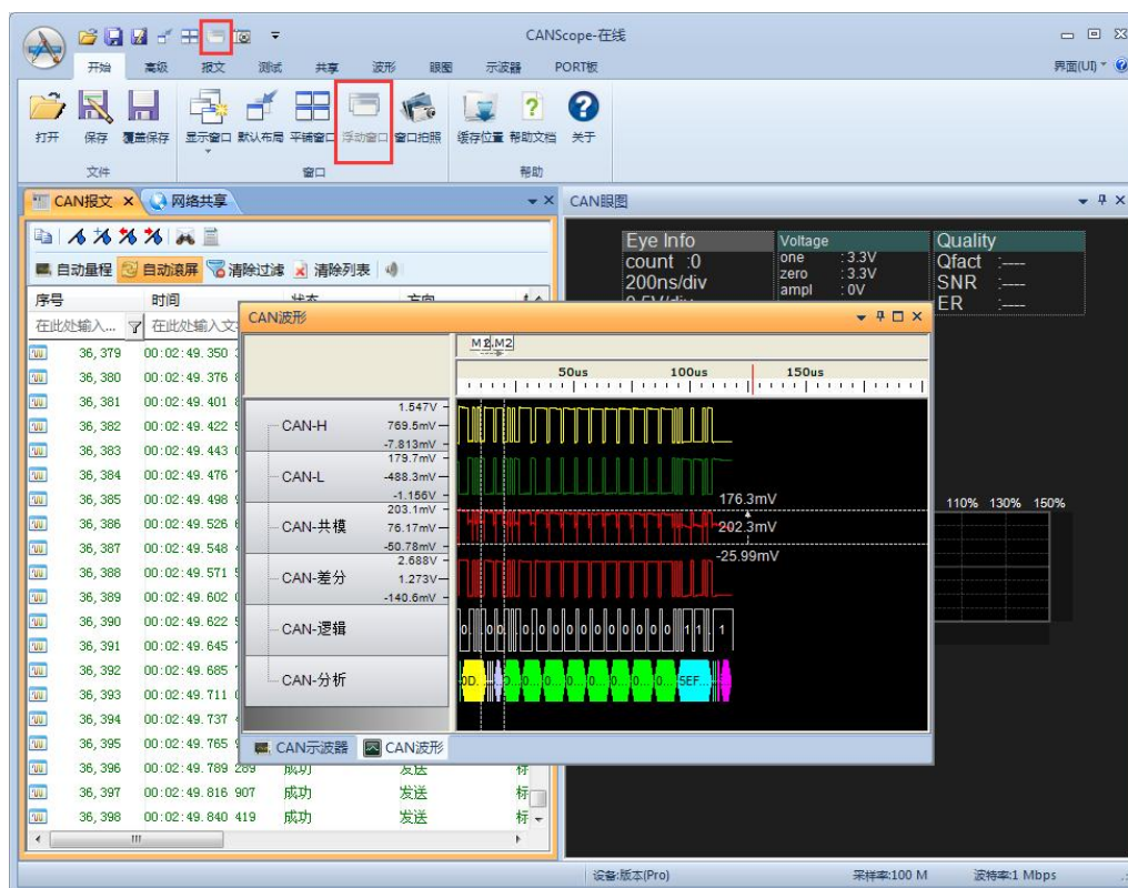
图 6.6 浮动窗口
