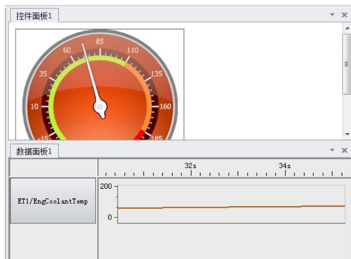
图 8.193 连接运行
