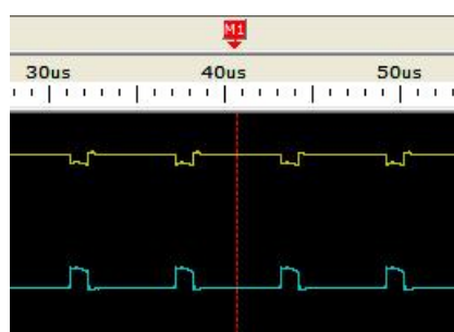
图 8.57 重叠的标签
