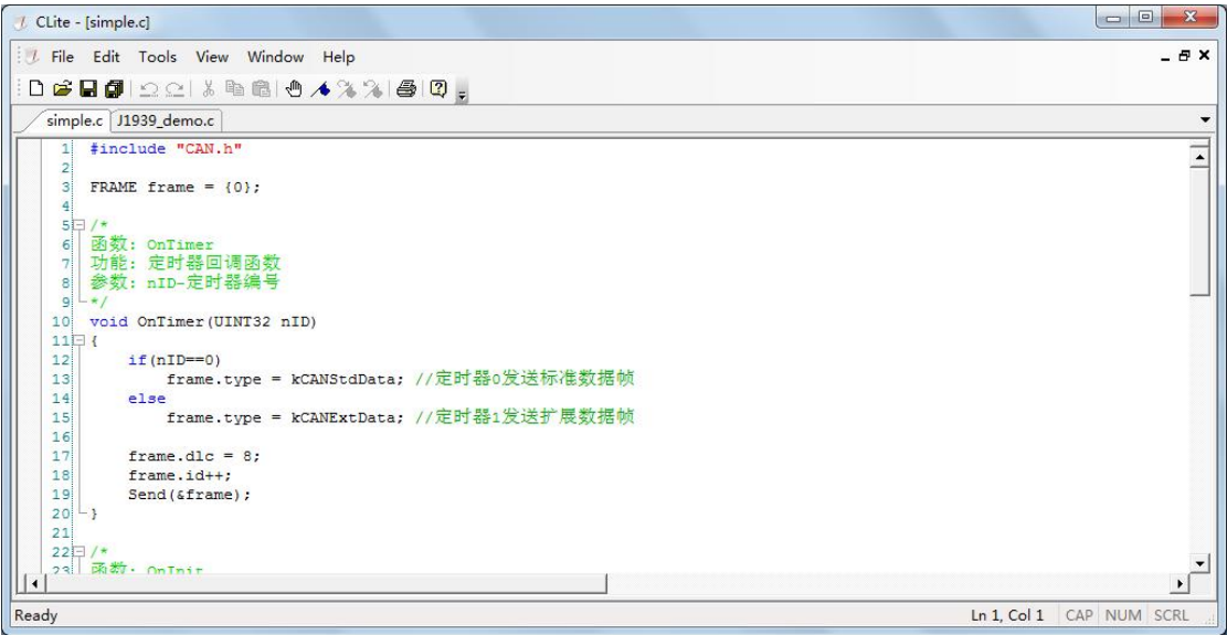
图 8.222 脚本模板
