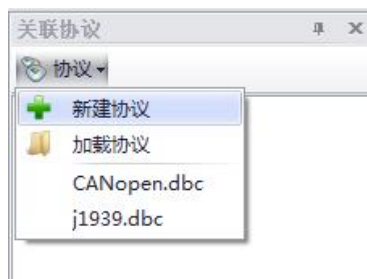
图 8.196 新建协议
