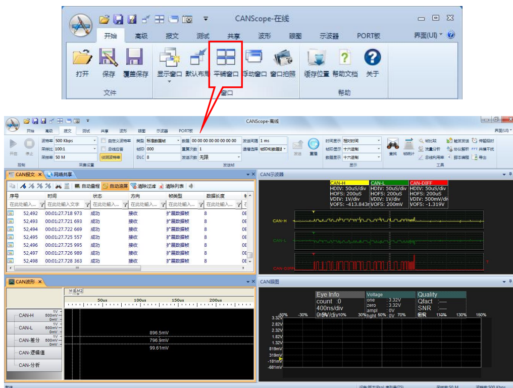
图 6.5 平铺窗口
