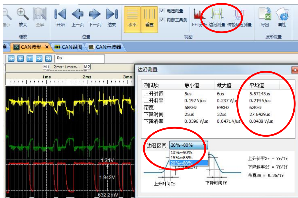
图 8.84 边沿测量
