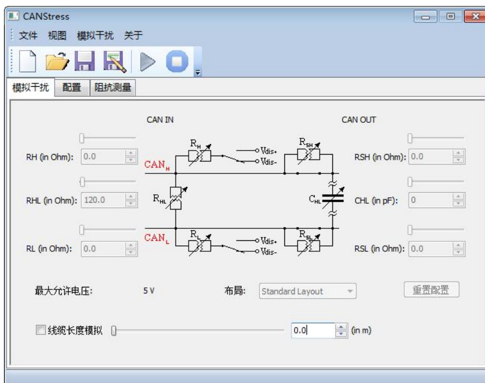
图 8.89“CANStress”窗口
