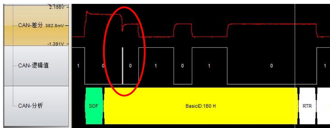
图 8.172 ID 仲裁的风险
