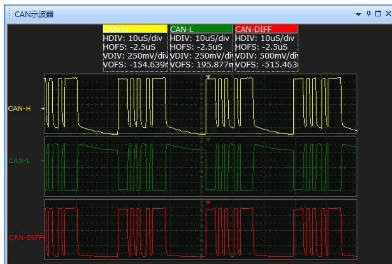
图 8.95CAN 示波器_ R HL (1300 欧姆) 测试结果
