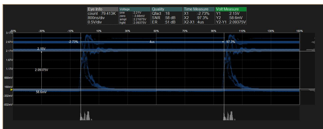
图 8.32 眼图轮廓效果
