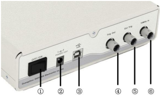
图 3.3 接线端
