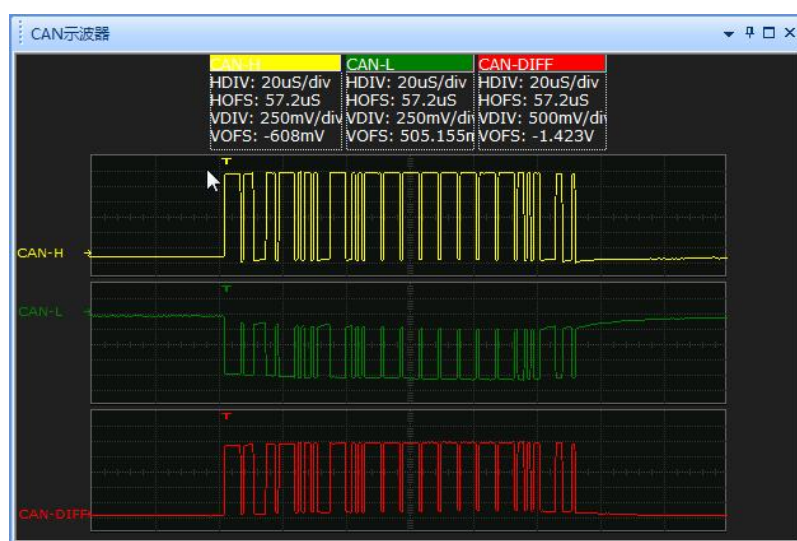
图 8.99CAN 示波器_ CHL (1000pf) 测试结果
