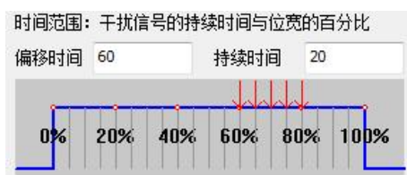
图 8.131 干扰位置
