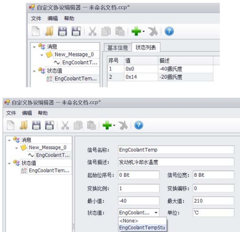
图 8.204 自定义协议_状态值设定 2
