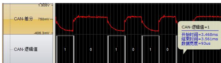
图 8.82 斜率过小导致波形畸变
