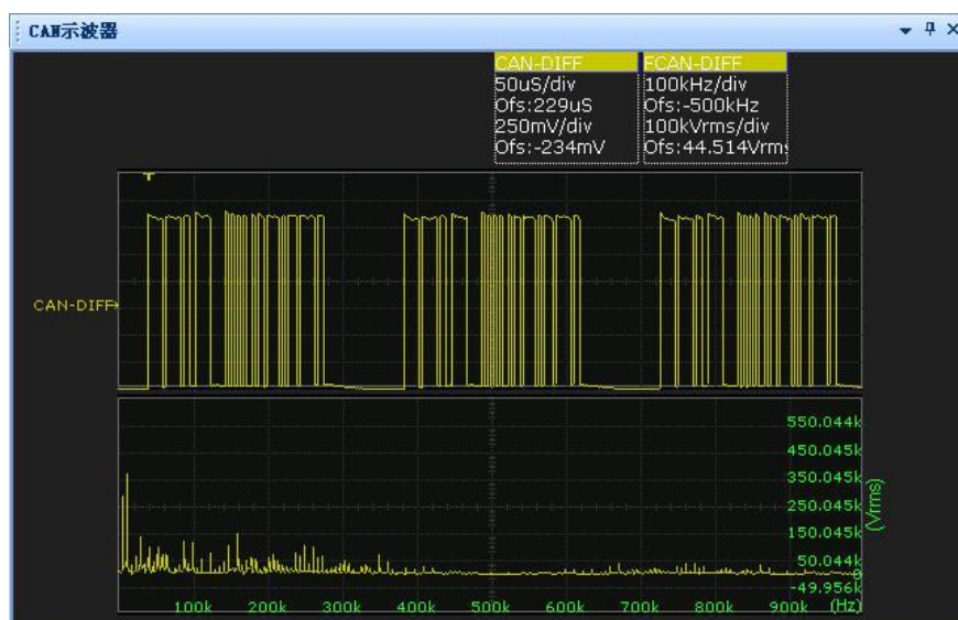
图 8.66 无干扰频率的差分信号 CAN_DIFF 的波形及其 FFT 分析
