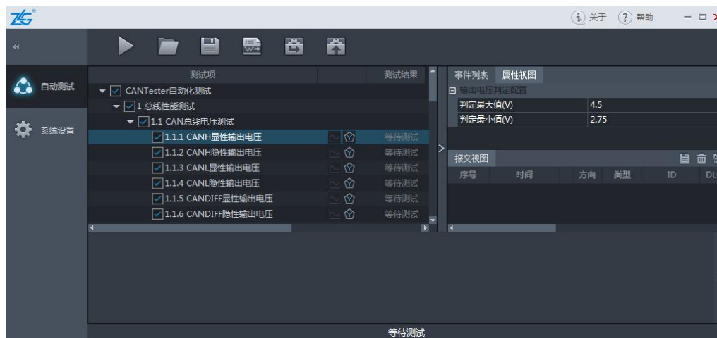
图 9.7 测试项选择
