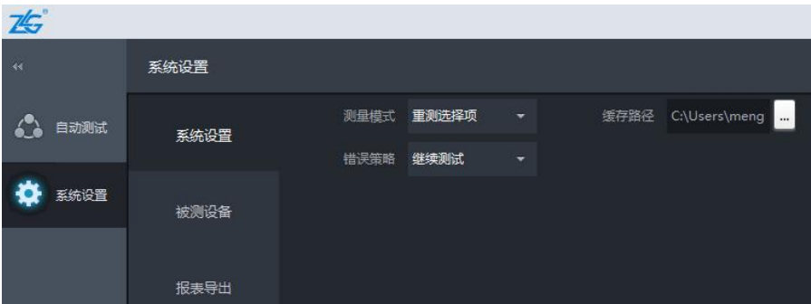
图 9.18 系统设置
