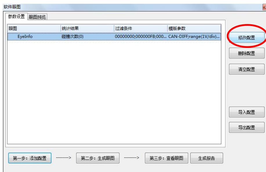
图 8.162 修改配置
