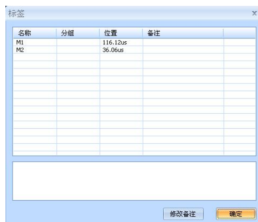
图 8.55 标签窗口
