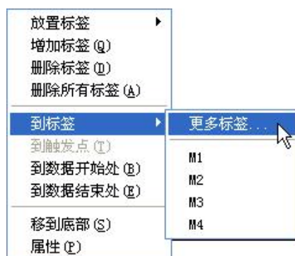
图 8.56 “到标签”命令
