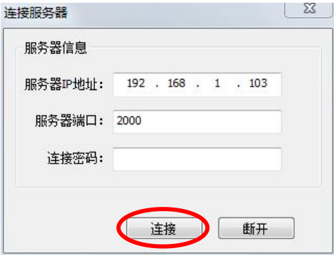
图 8.181 连接服务器
