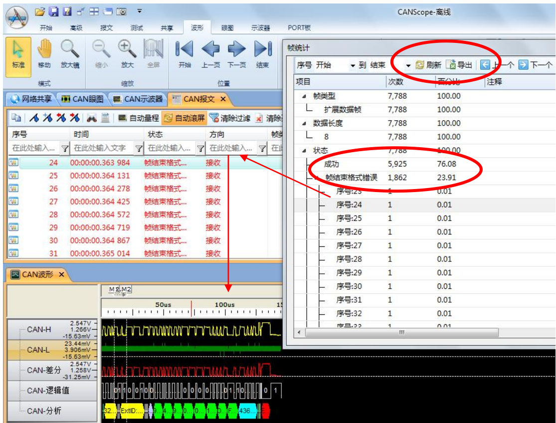
图 8.37 帧统计框
