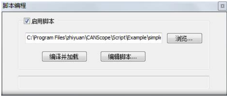
图 8.221 脚本编程
