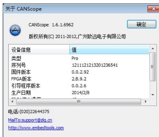
图 6.8 “关于”窗口
