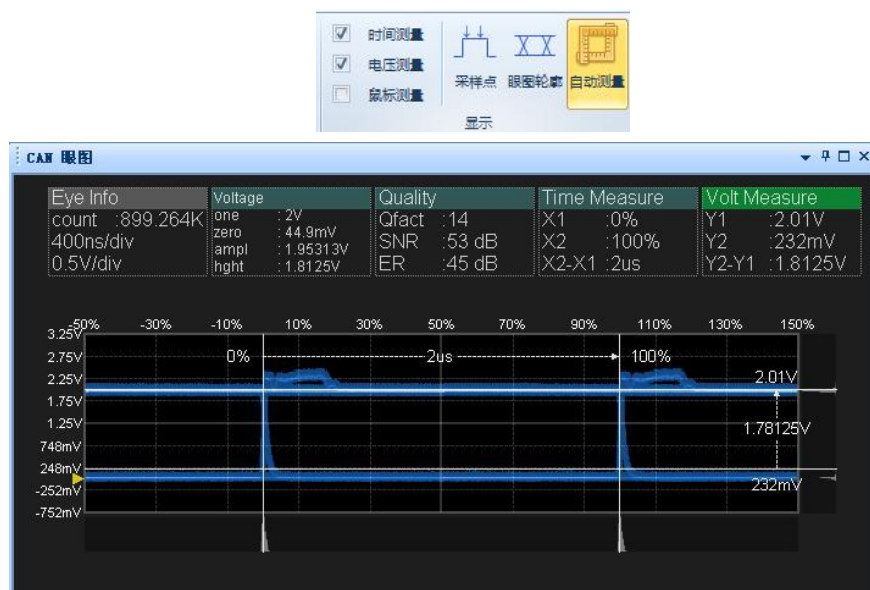
图 8.29CAN 眼图_时间测量和电压测量
