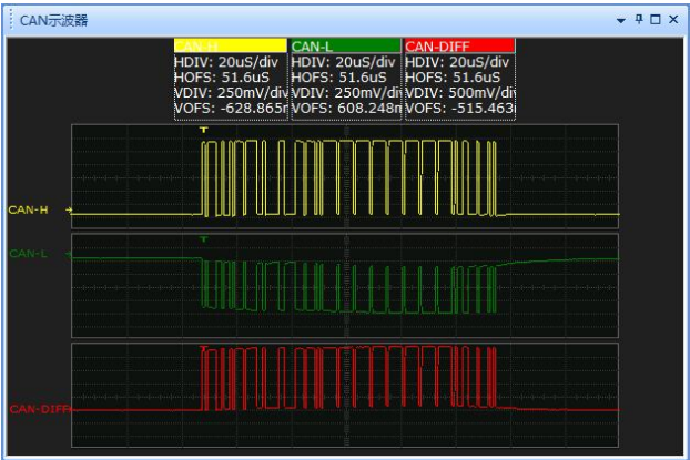
图 8.93“CAN 示波器”_R_HL（120 欧姆）测试结果
