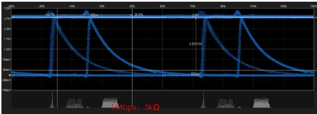
图 8.97 终端电阻过大
