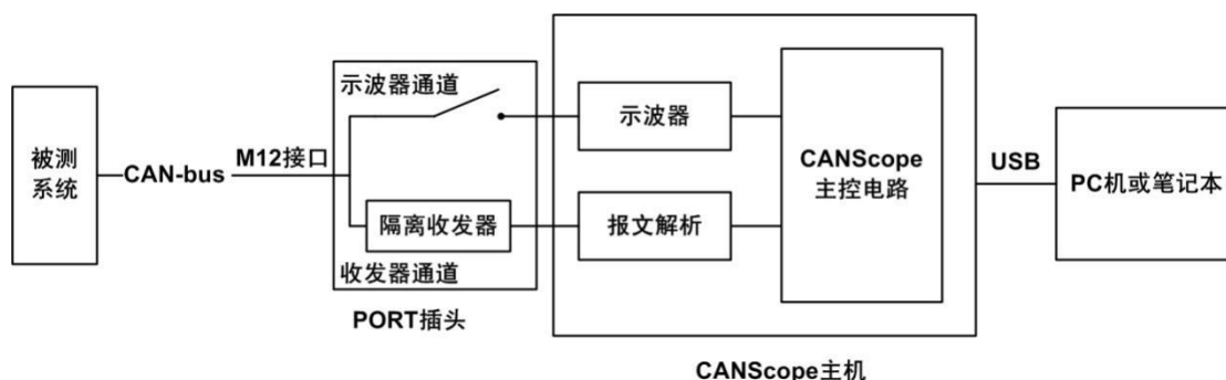
图 3.1 系统连接示意图
