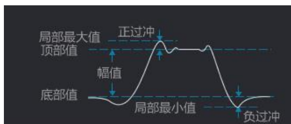
图 3.6 过冲判定
