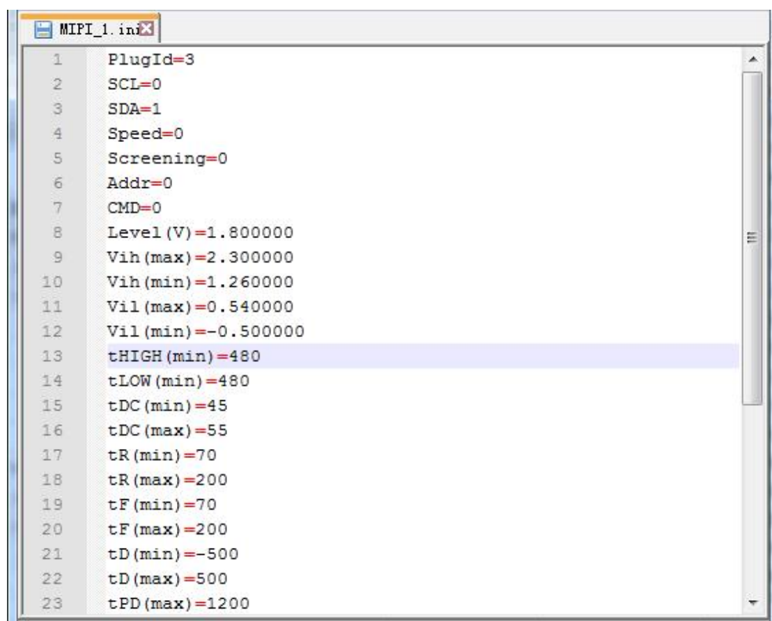
图 4.1 ini 文件格式(ZDS4000/5000 系列示波器)
