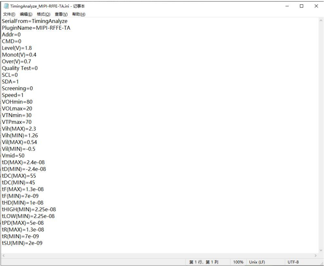
图 4.2 ini 文件格式(ZUS6000 系列示波器)
