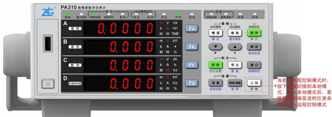
图 1.1 前面板相关按键
