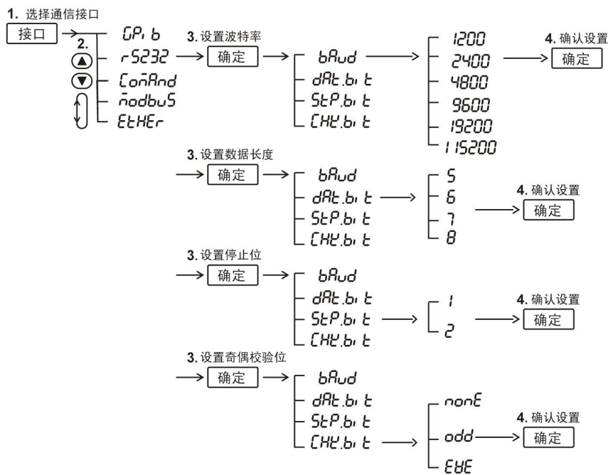
图 3.4 RS-232 接口设置流程
