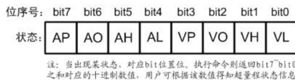
图 7.2 过量程状态编码
