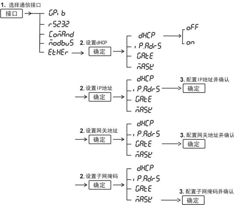
图 4.4 Ethernet 接口设置流程
