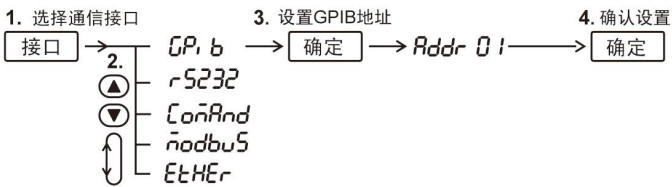
图 2.4 GPIB 设置流程
