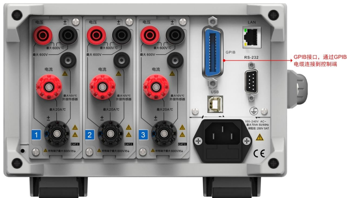
图 2.3 PA323/PA333H/PA323H 型功率计 GPIB 接口
