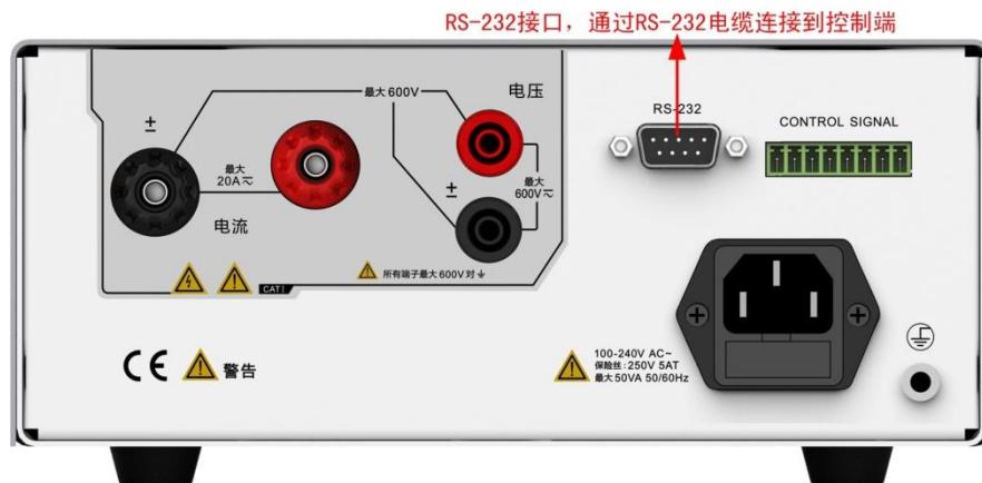
图 1.2 RS-232 接口
