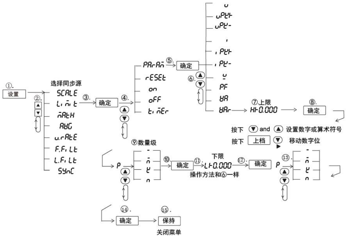
图 11.5 侦测参数设置流程
