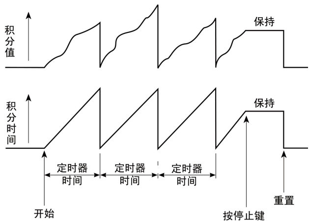
图 10.4 连续积分模式
