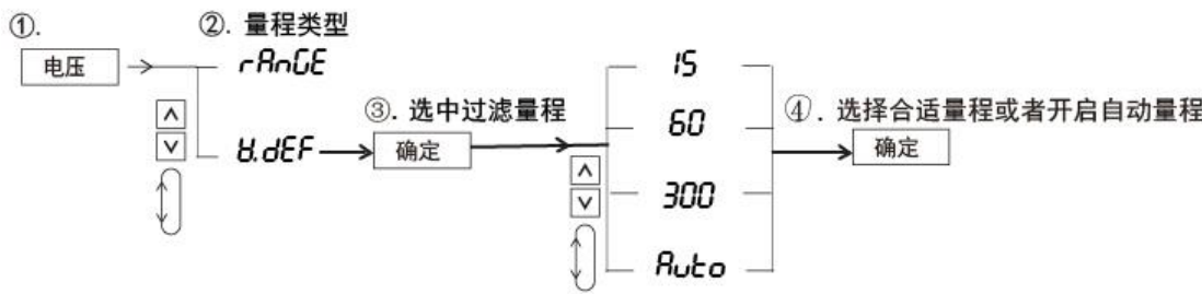
图 12.16 使用电压量程过滤表
