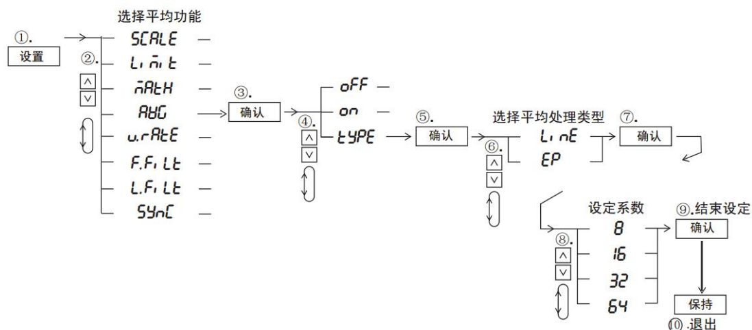
图 6.16 平均功能操作流程示意
