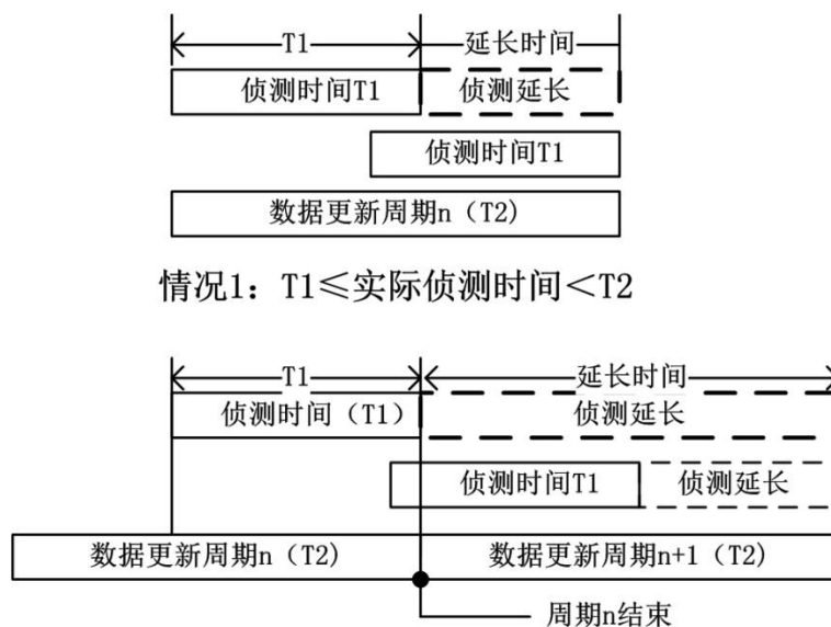
图 11.9 侦测时间小于数据更新时间情况
