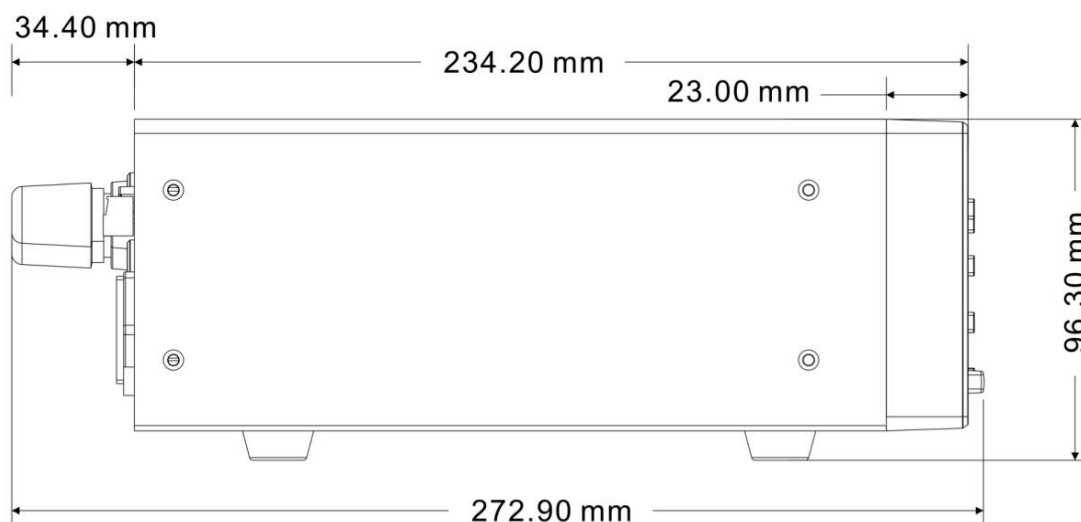
图 15.2 PM100 型功率计机械尺寸图（侧面）
