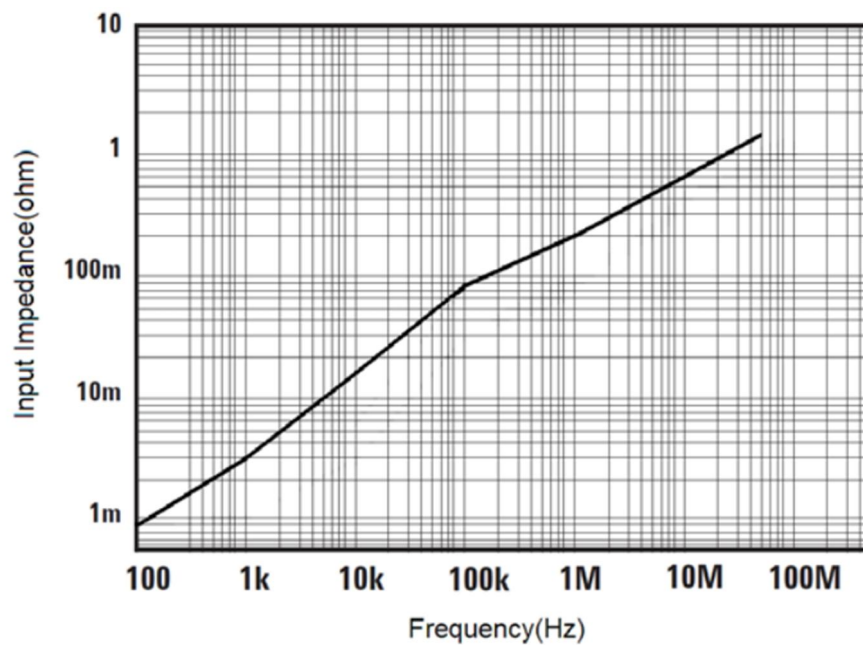
图 5 ZCP30 输入阻抗 VS 测量频率
