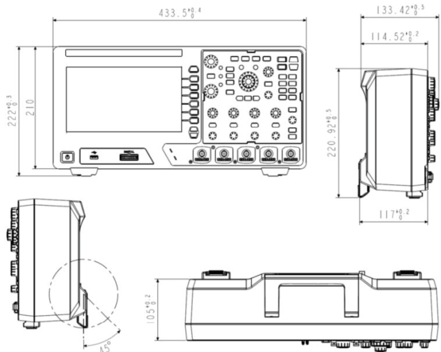
图 4.1 ZDS2000C 示波器尺寸图
