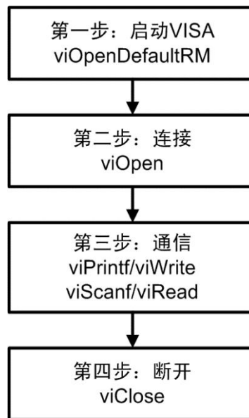
图 22.3 VISA 通信流程步骤
