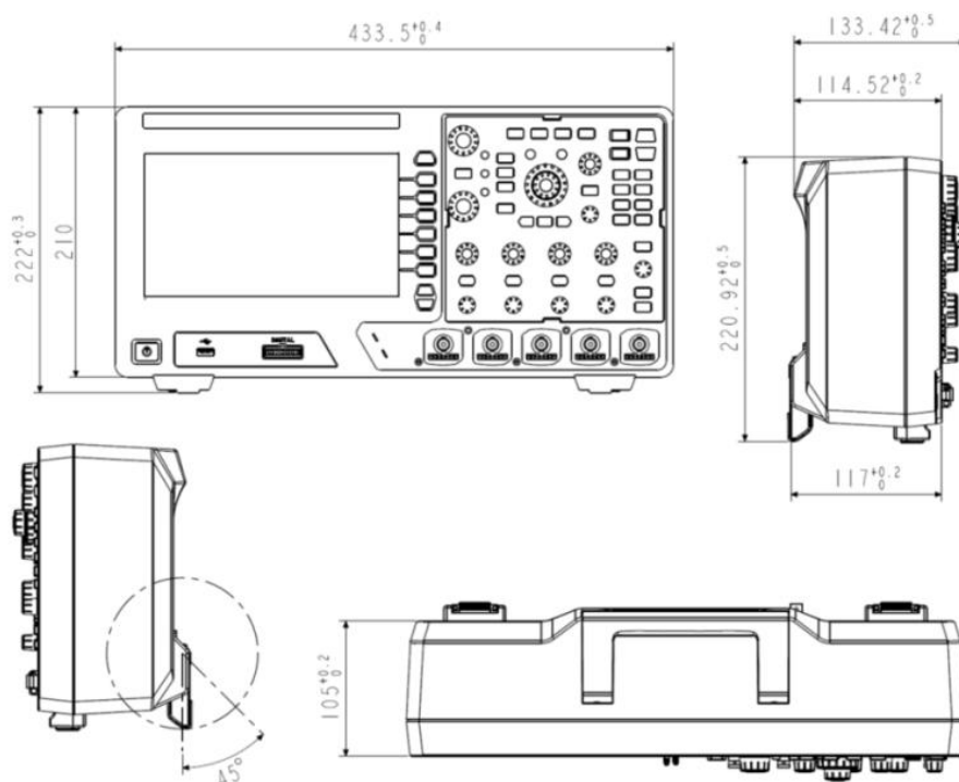
图 4.1 ZDS3024C 示波器尺寸图
