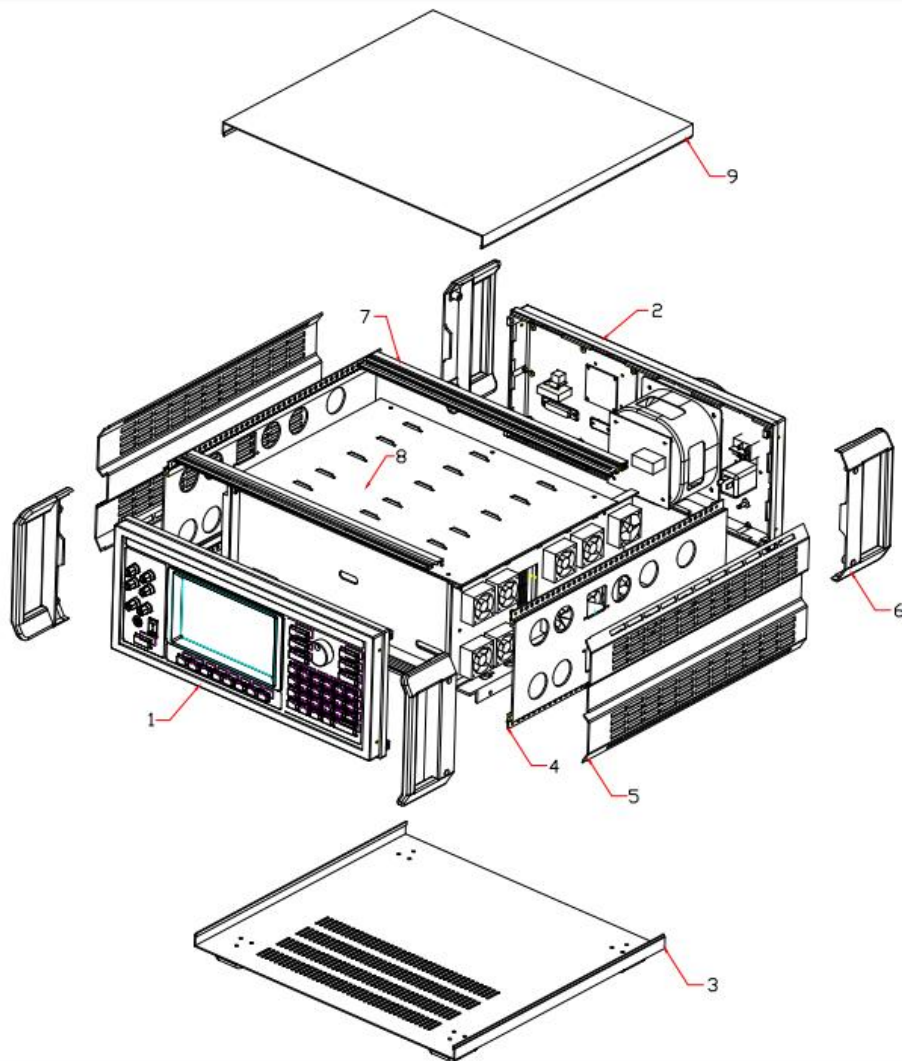
图 2.4 整体结构图
