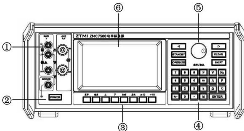
图 2.2 前面板示意图
