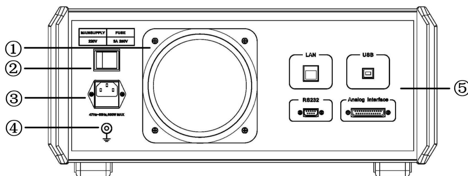
图 2.3 后面板示意图
